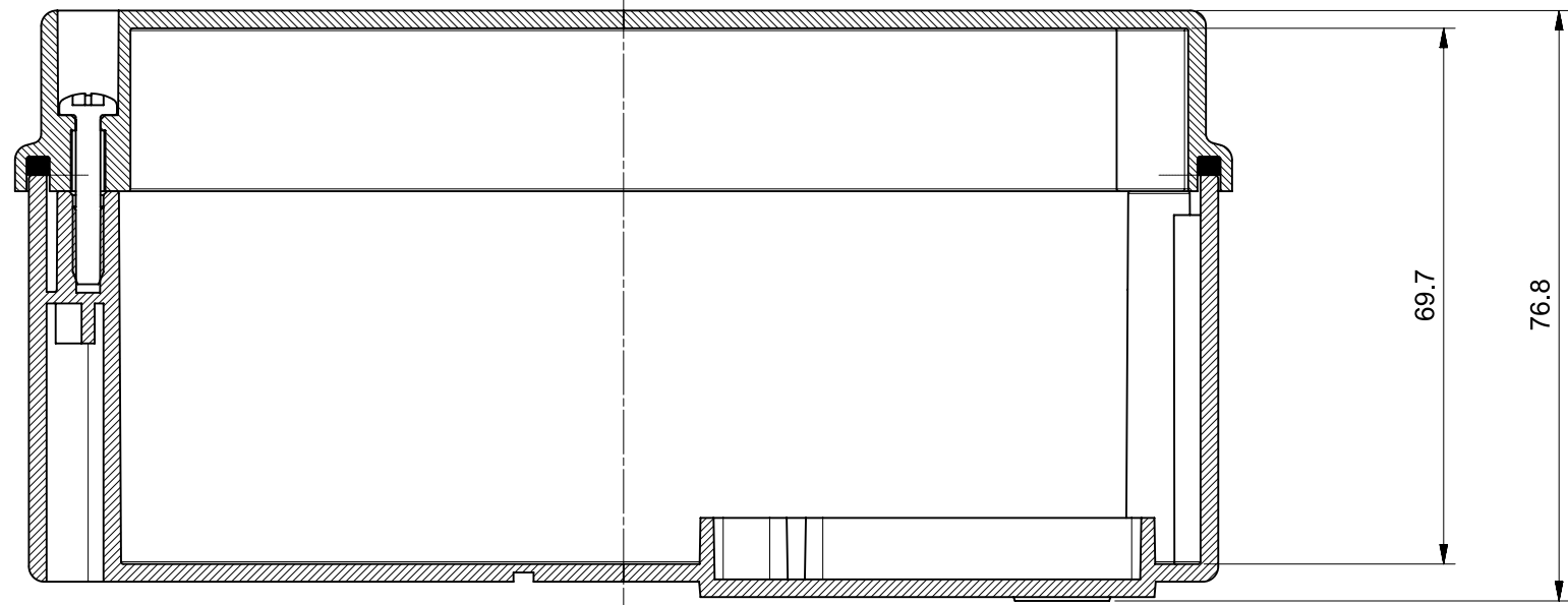
Sezione A-A
