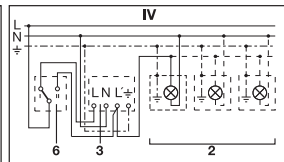
4. Aansluiting via een wisselchakelaar voor permanente verlichting en automatische werking Stand I: automatische werking Stand II: handschakeling voor permanente verlichting Opgelet: Uitschakelen van de installatie is niet mogelijk, alleen de keuze tussen stand I en II.
