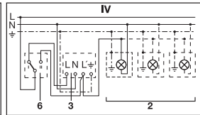
Anslutning via trappströmställare för permanent ljus resp. sensorstyrd drift Läge I: Sensorstyrning, av/på styrs av sensorn Läge II: Manuell drift, permanent belysning Observera: Frånkoppling av anläggningen är inte möjlig, man kan endast välja mellan läge I och läge II.
