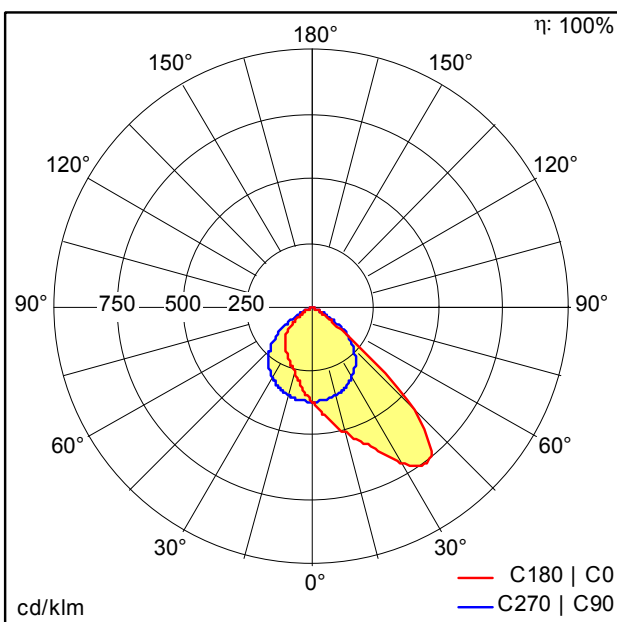
TE_LEO_FLEX_80W_840_FLEX1.idt
